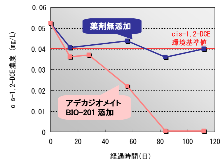
図6 汚染物質の分解挙動(ビーカーテスト)
