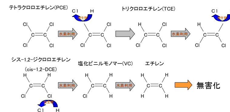
図5 分解経路
